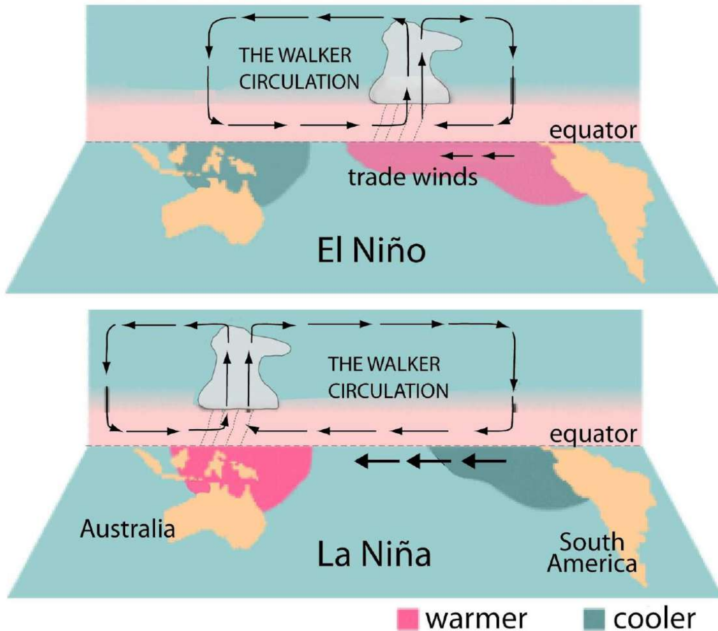
Fig. 1) Circulación atmosférica ecuatorial durante El Niño y La Niña
