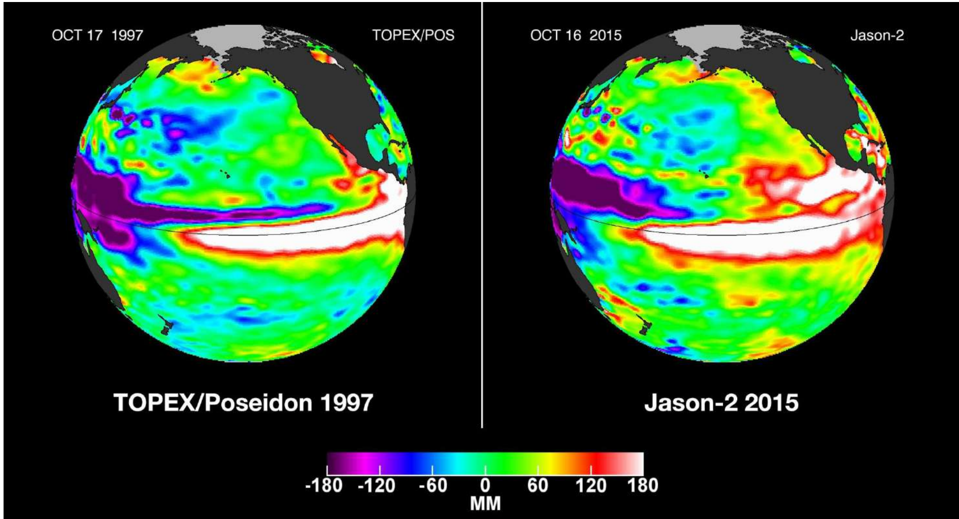
Fig. 1) Anomalía del Nivel del Mar, El Niño en octubre 1997 y 2015 (NASA-JPL , 2015)
